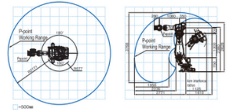
FD- V350
