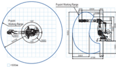
FD- V400L
