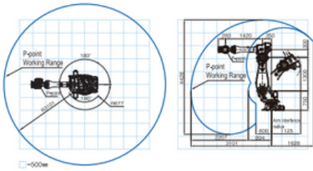
FD- V280L
